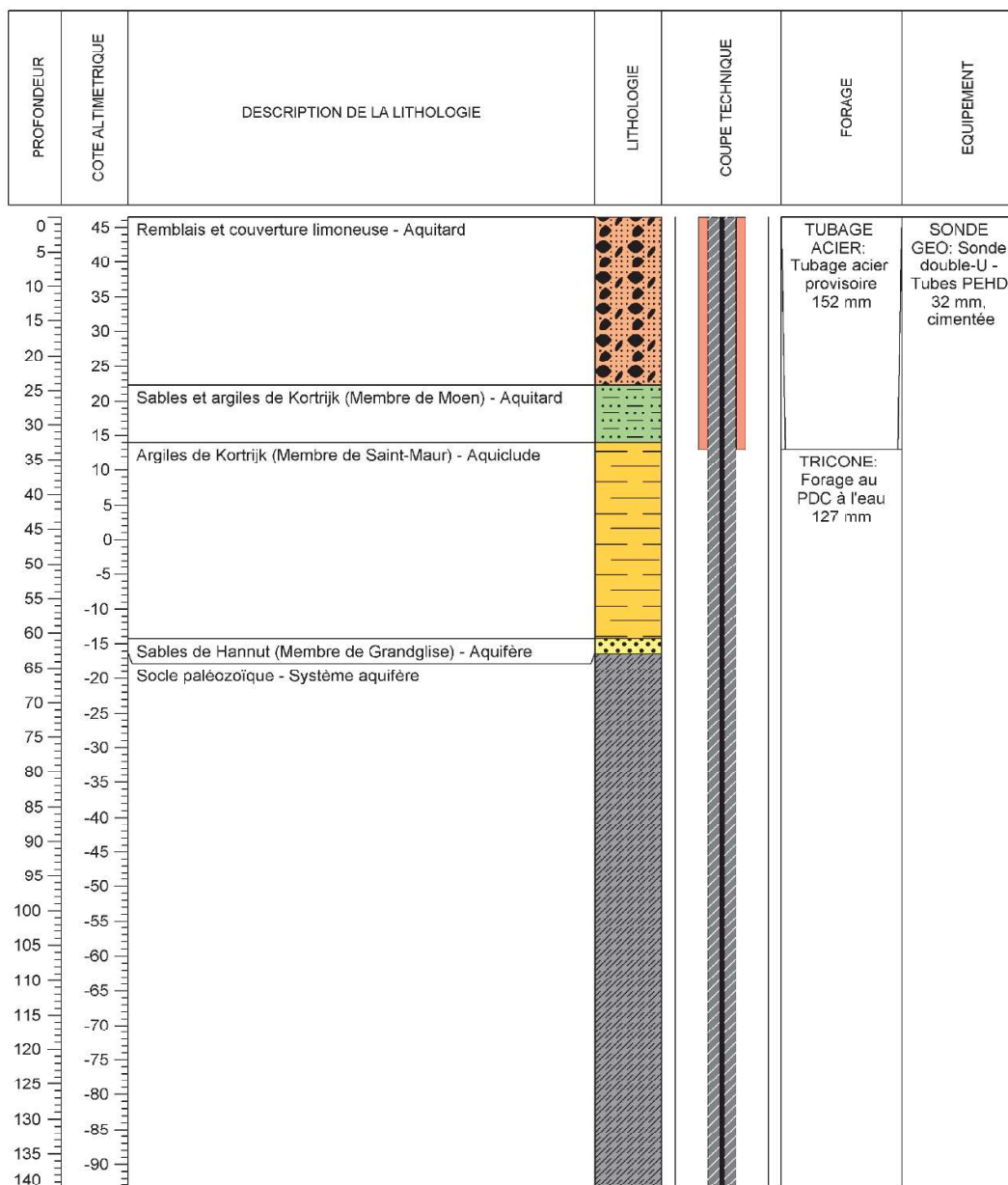
Figure 3-1 : Coupe prévisionnelle de la sonde géothermique test
