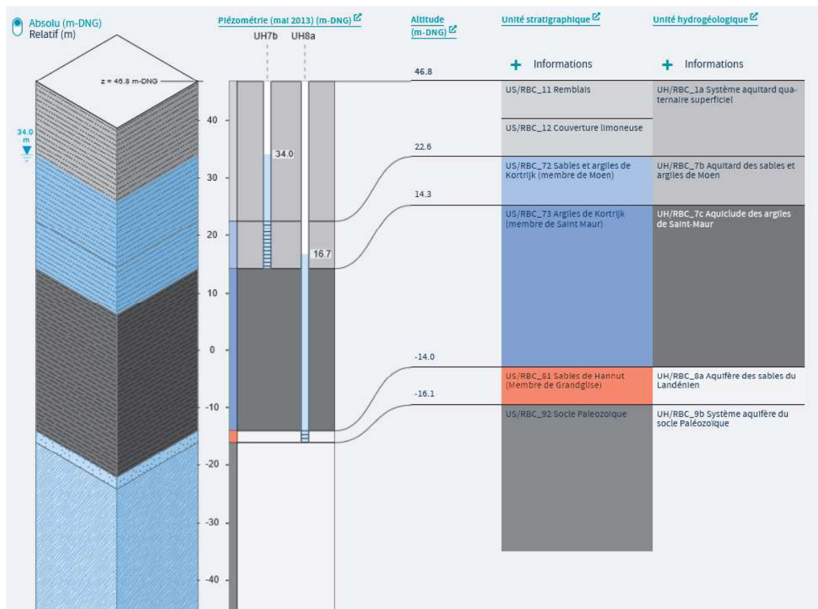
Figure 1-1 : Forage virtuel au droit du site 1
